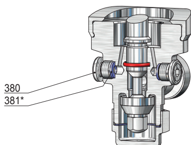
Manometerbohrung G ¼
