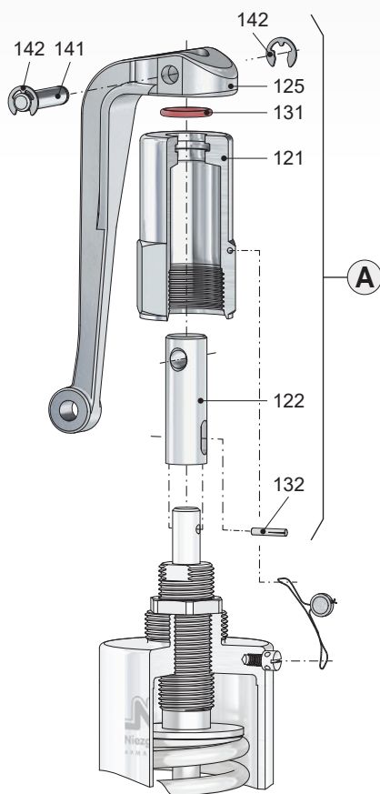
Ventilkopf A
