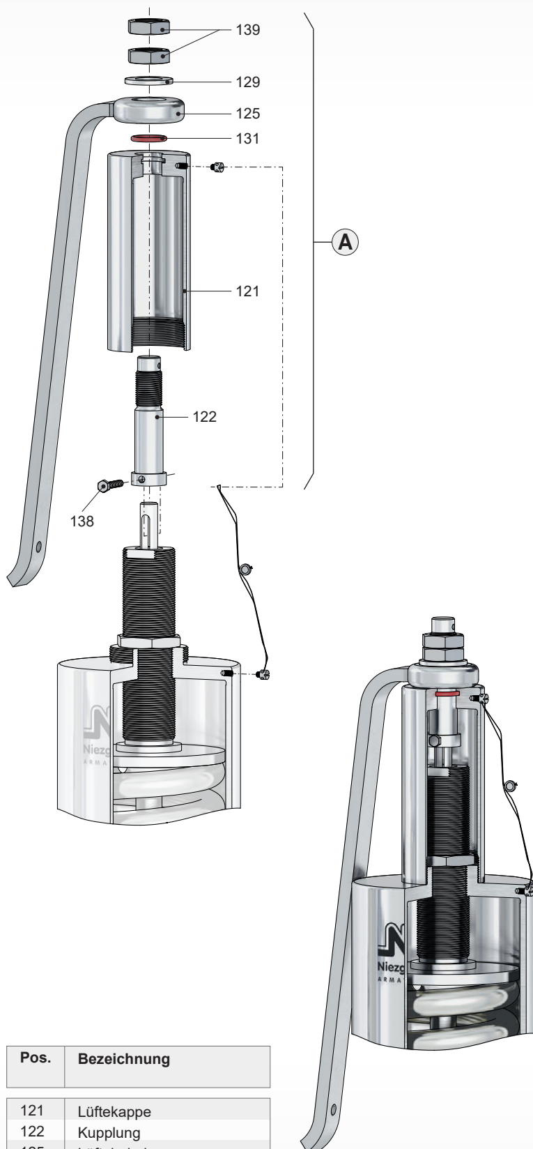
Ventilkopf A
