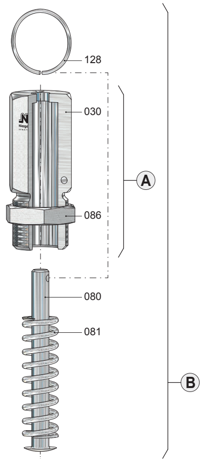
Ventilkopf D
