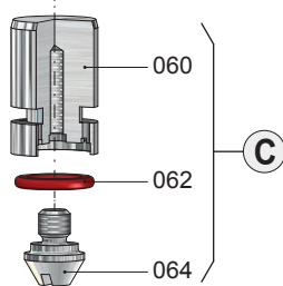
Kegel mit O-Ring
