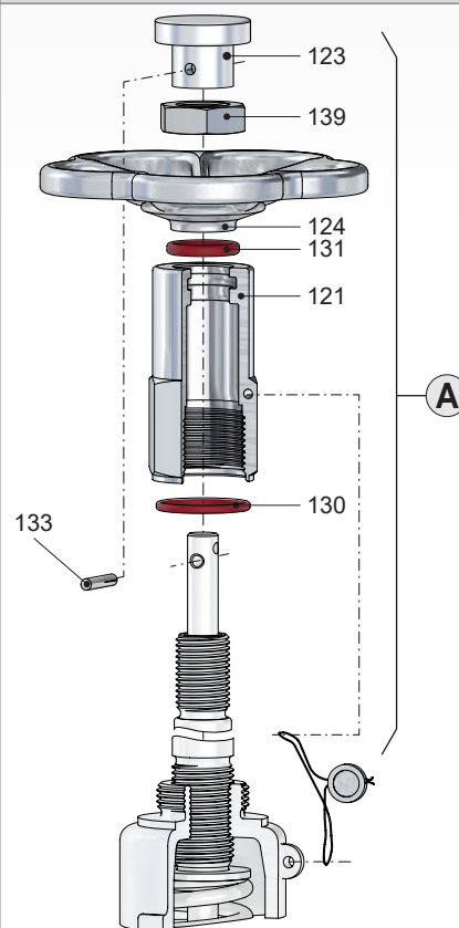
Ventilkopf G
