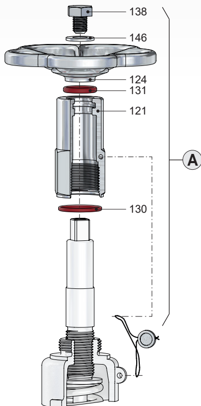
Ventilkopf F
