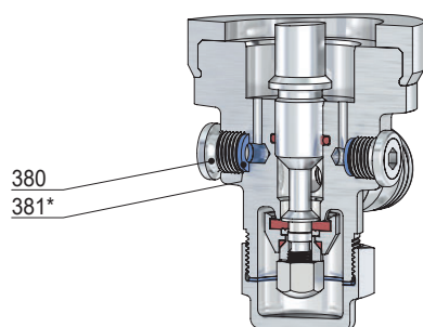
Manometerbohrung G 1/4
