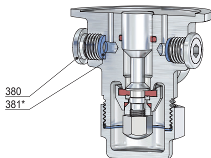
Manometerbohrung G 1/4
