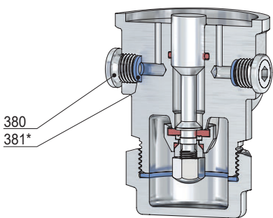
Manometerbohrung G 1/4
