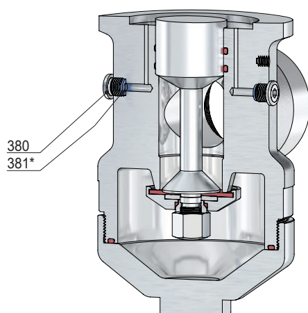
Manometerbohrung G 1/4
