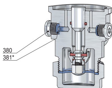
Manometerbohrung G 1/4
