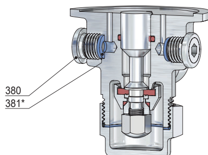
Manometerbohrung G 1/4
