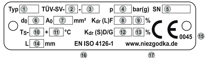
Abbildung 2: Typenschild nach DIN EN ISO 4126
